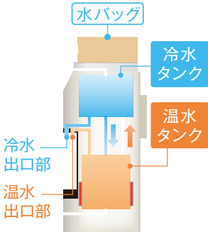
高温循環システム イメージ図
